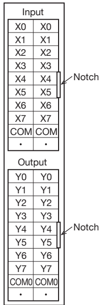
FX5-C32ET/D
