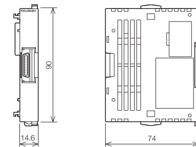
FX5-CNV-IFC
